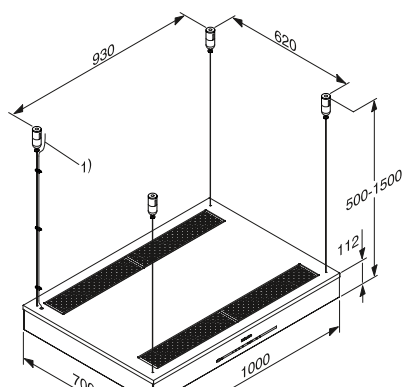
DA 6700 D - Island
