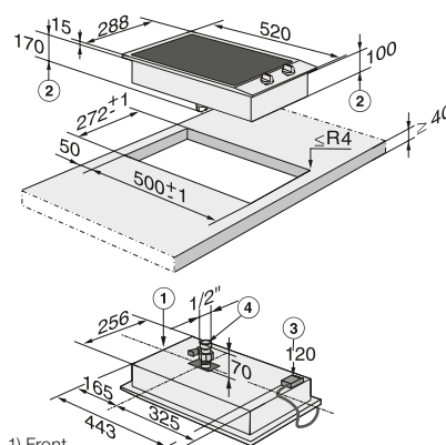
Grill CS 1312 BG
