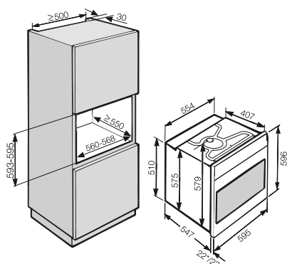
H 6461 BP, H6860 BP, 76 l cavity
