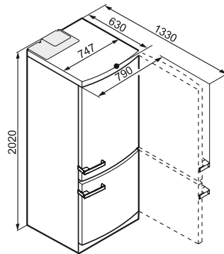
KFN 14947 SDE ed
