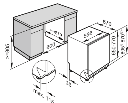
G 6260 Scvi, G 4960 Scvi
