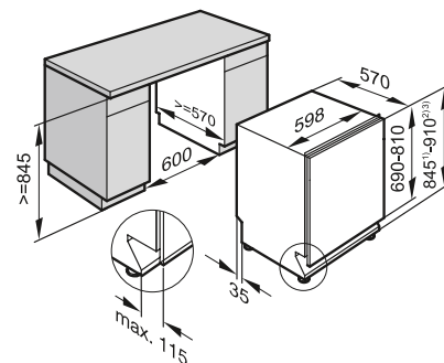
G 6995 Scvi XXL
