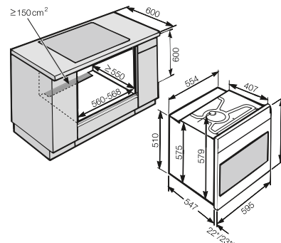
H 6461 BP, H6860 BP, 76 l cavity
