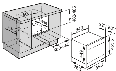
DGC 6800 XL, 48 l cavity
