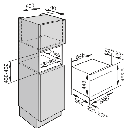
DGC 6800 XL, 48 l cavity
