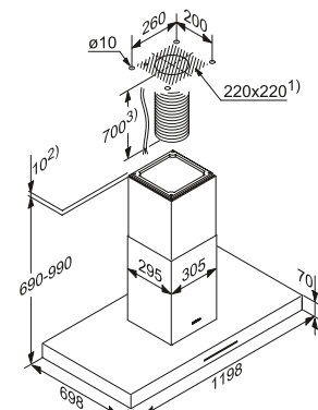
DA 424 V-6 - Island
