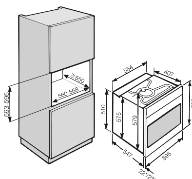
H 6260 B, 76 l cavity
