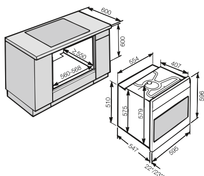
H 6260 B, 76 l cavity
