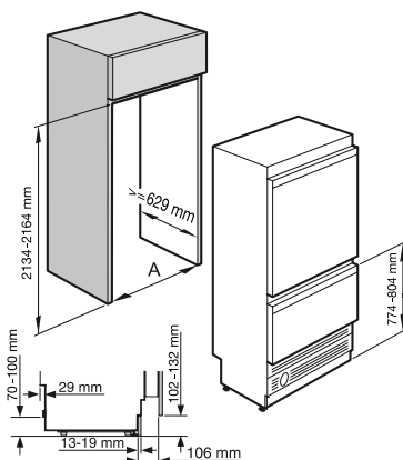
KF 1901 Vi, KF 1911 Vi
