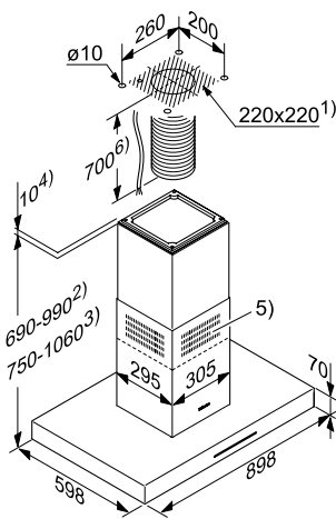
DA 410-6-D - Island
